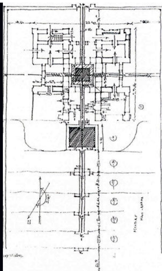
پلان باغ و کوچه چشمه عمارت. ترسیم از هانری ویوله ۱۴-۱۹۱۳ م. Mrs. Marine Fromanger ماسخند:
